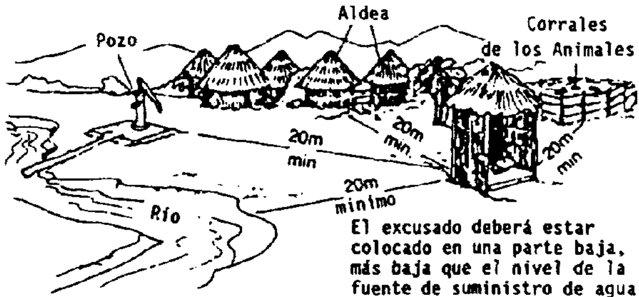
Figura 1. Ubicación Correcta del Excusado
